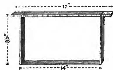
FIG. 14.—Standard Frame.
